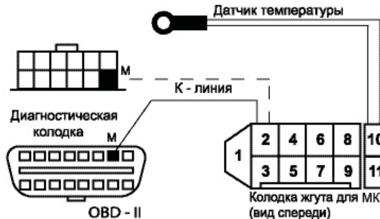
Рис. 1. Подключение МК.
