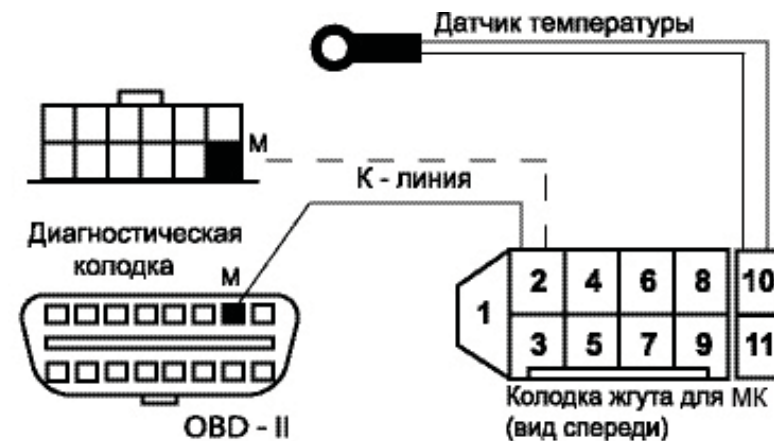
Рис. 1. Подключение МК.
